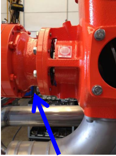
Sichtfenster Dichtungskontrolle
